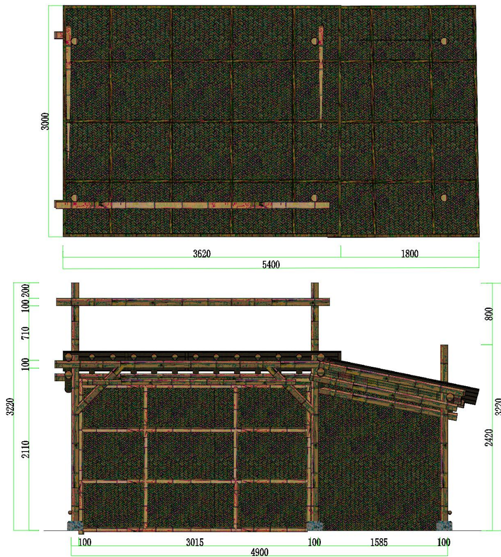
帝师桥 摊位C款 数量4组 钢木结构
