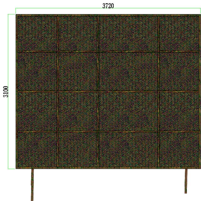
帝师桥 摊位D款 数量4组 钢木结构
