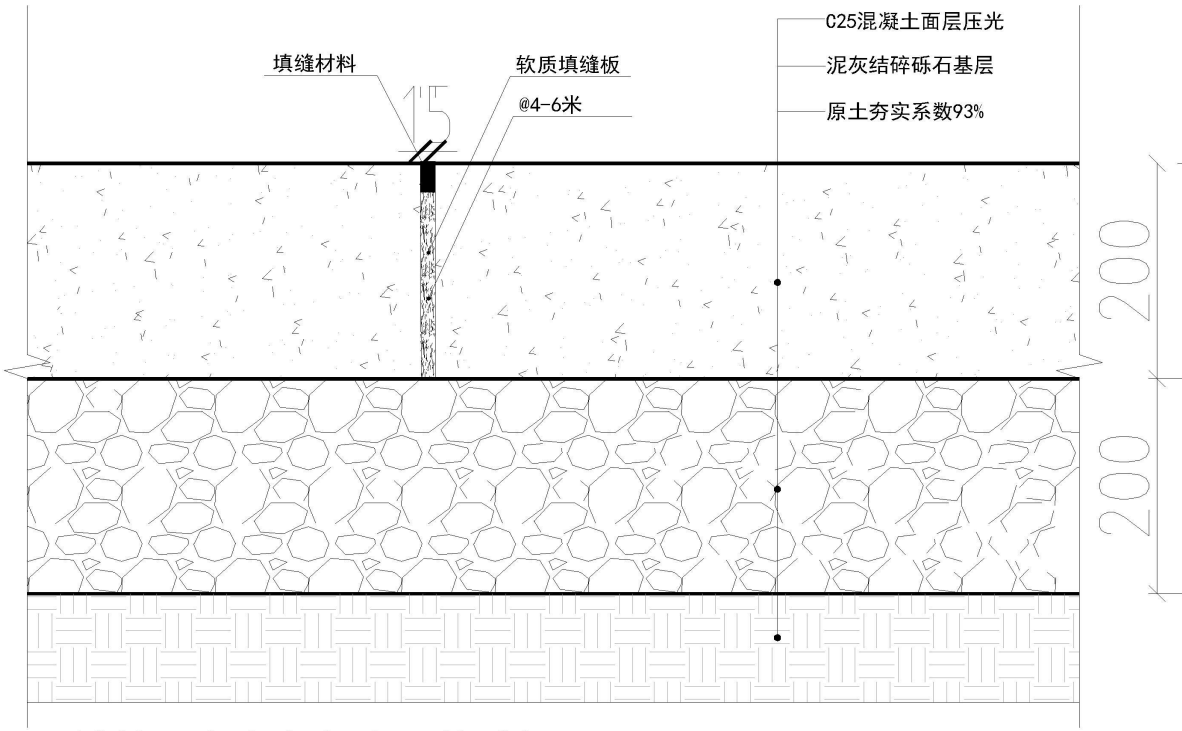
天桥社区山水名都小区篮球场 原有地面300x600x50mm青石板及水泥砂浆粘接层（50mm）拆除 新做篮球场地面剖面图
