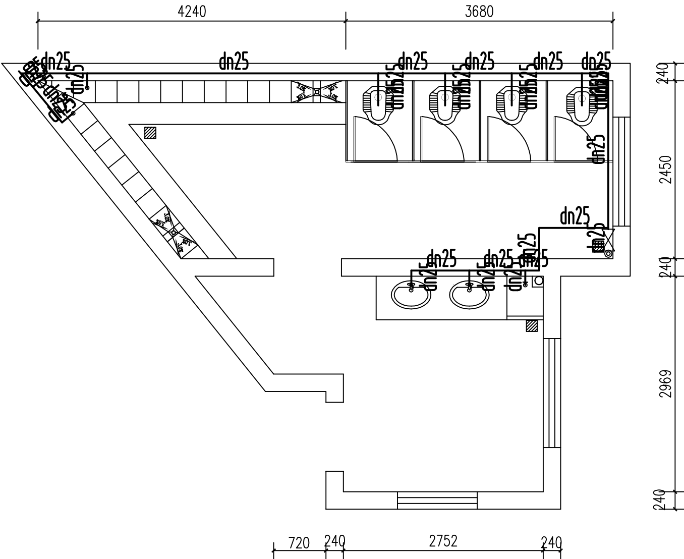
尚雅楼男卫生间给水线路图 1:50
