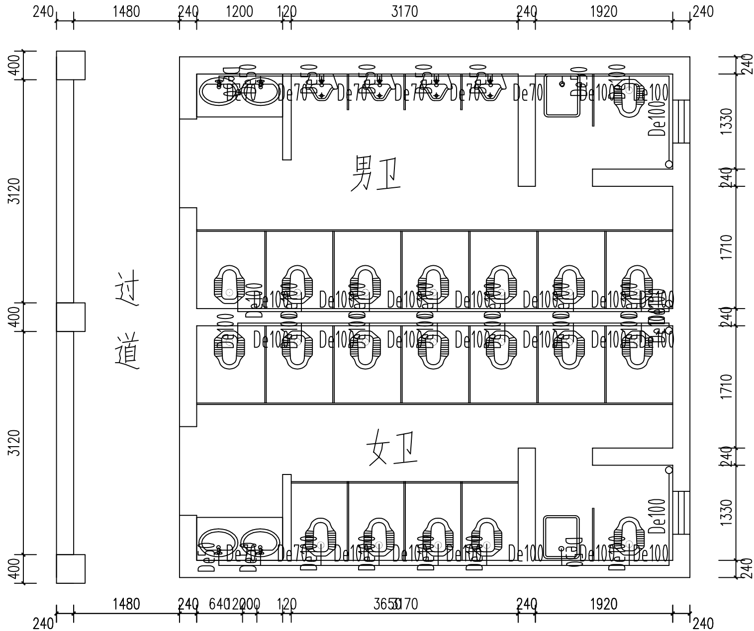
五楼男、女卫排水线路图 1:50
