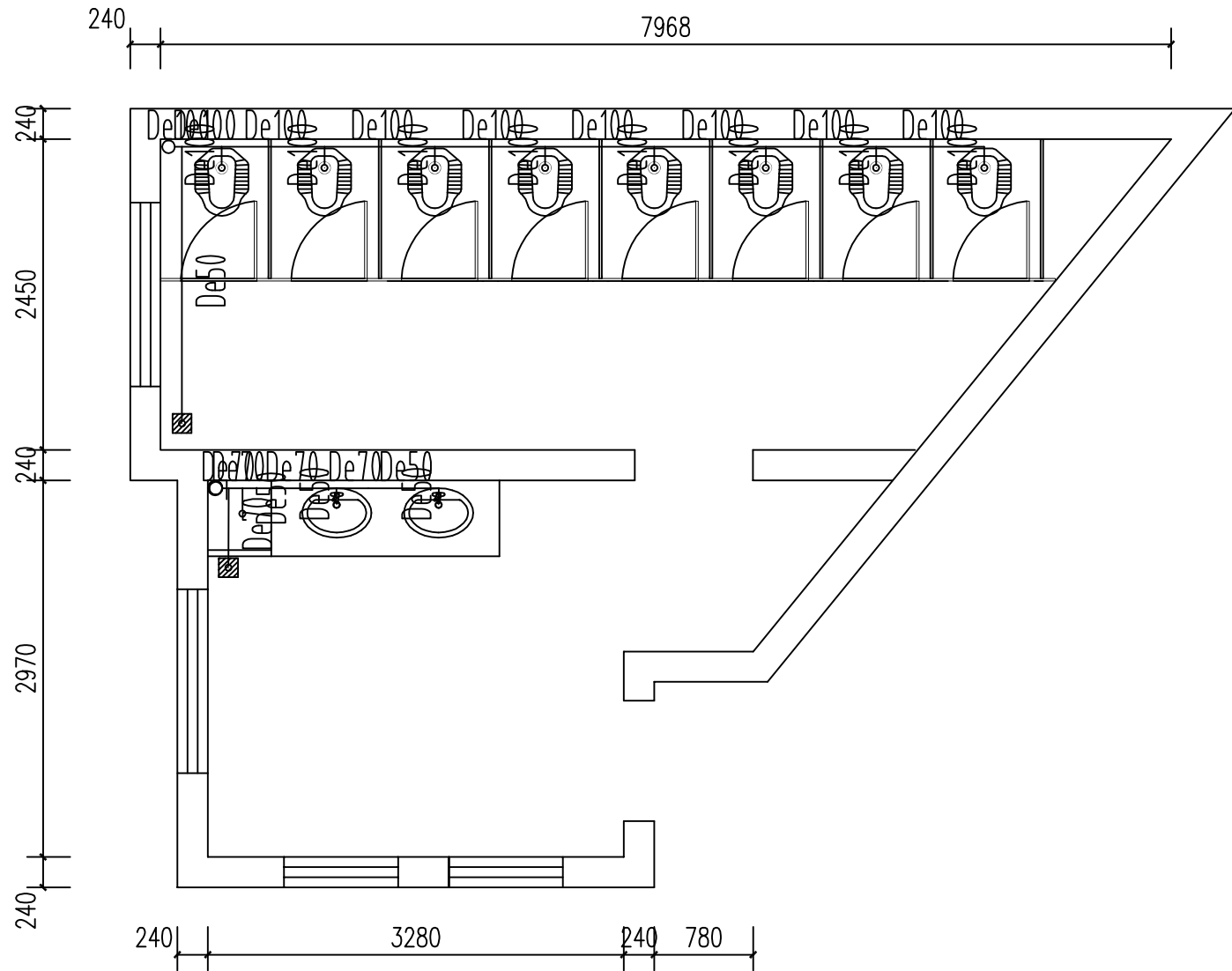
尚雅楼女卫生间排水线路图 1:50
