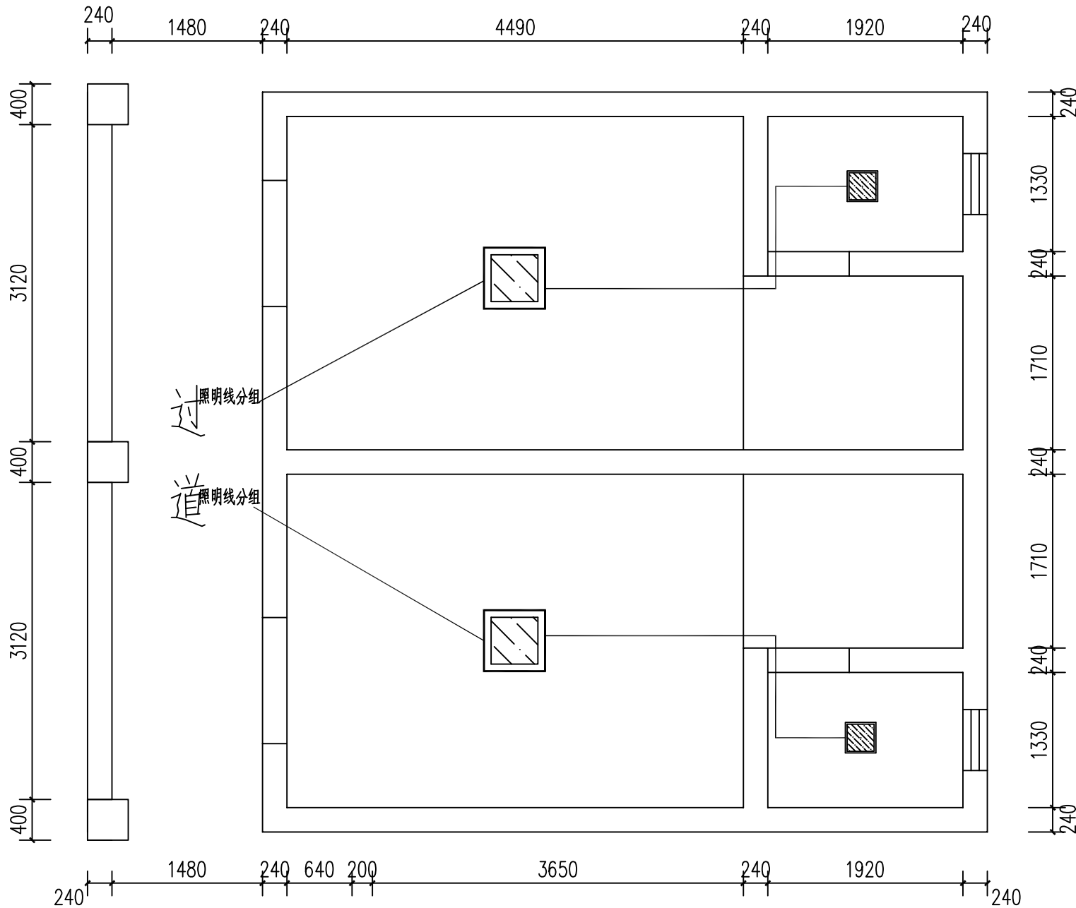
五楼男、女卫照明线路图 1:50
