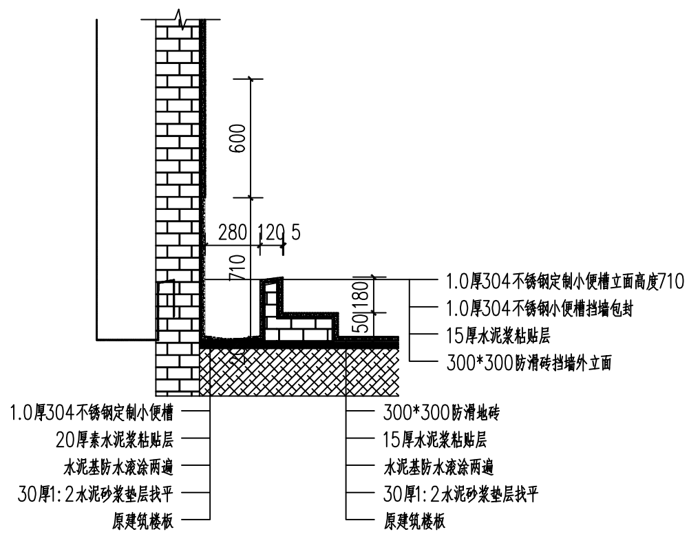
不锈钢小便槽剖面
