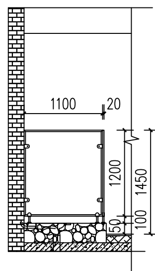
1-1剖面尺寸图
