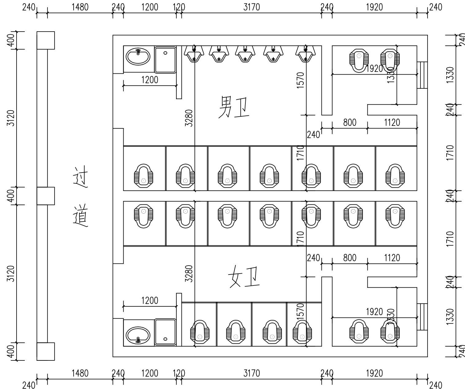
三原男、女卫平面图 1:50
