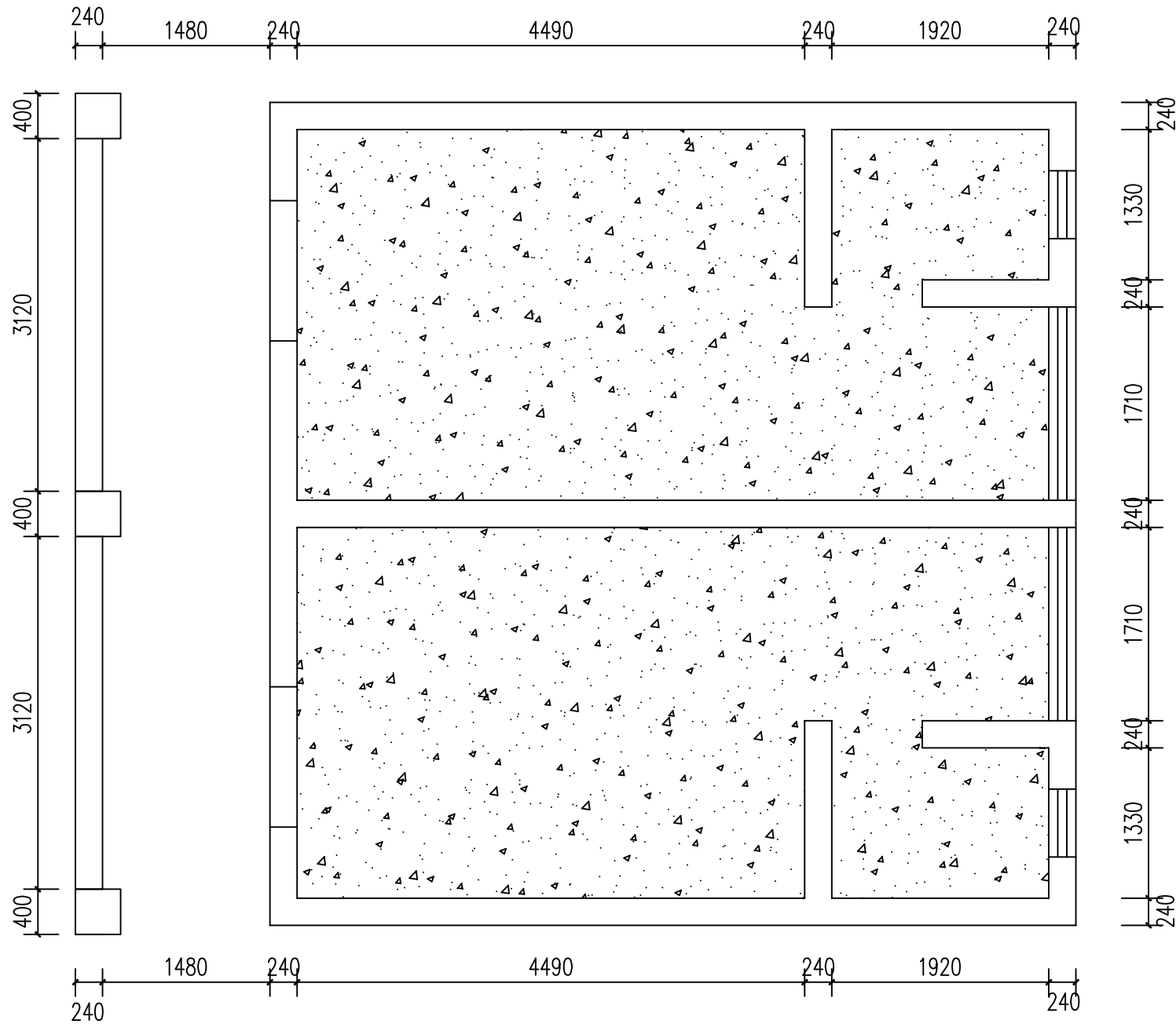
二楼监控室拆除范围 1:50
