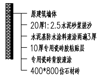
墙砖铺贴大样
