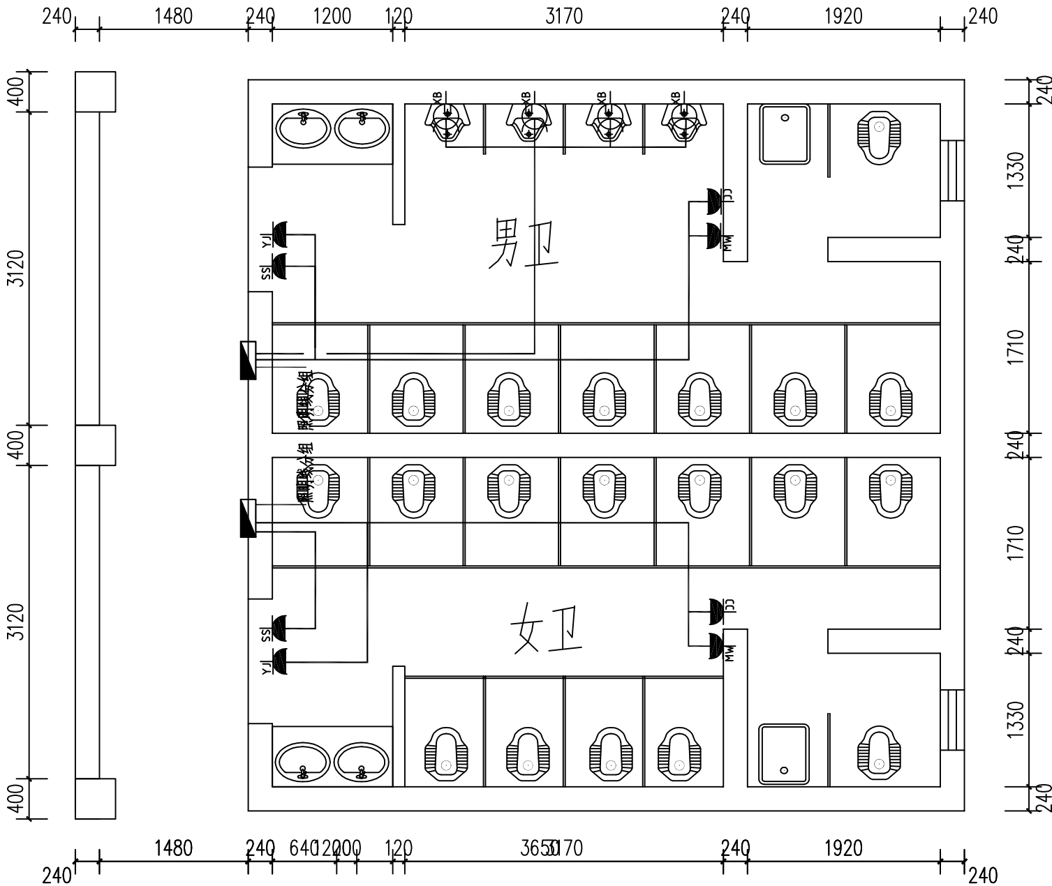
五楼男、女卫强电线路图 1:50
