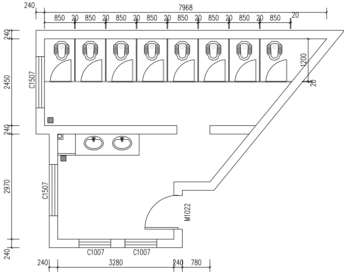
尚雅楼女卫整改平面图 1:50
