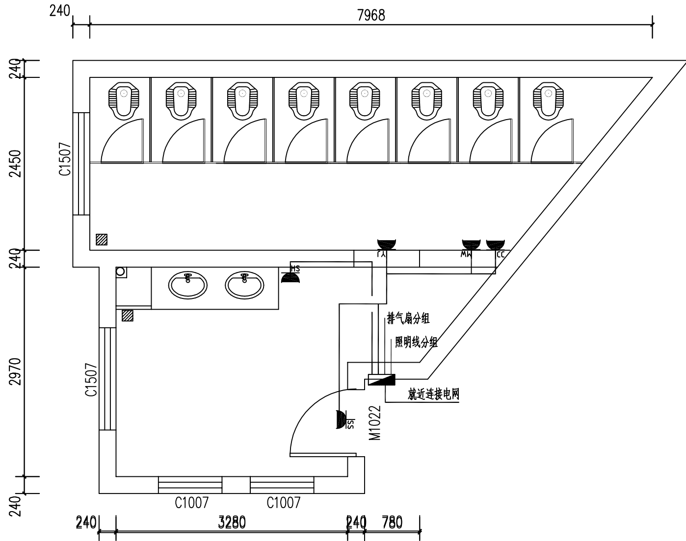
尚雅楼女卫生间强电线路图 1:50
