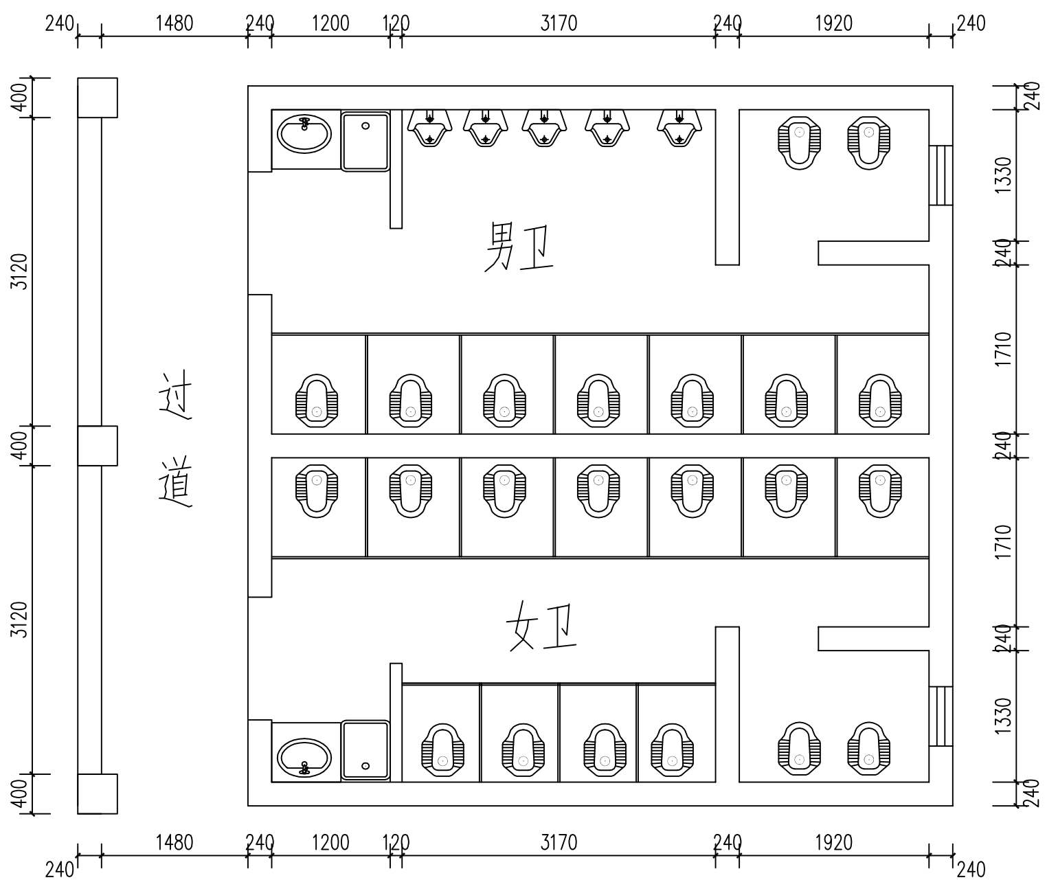
三楼男、女卫拆除范围 1:50
