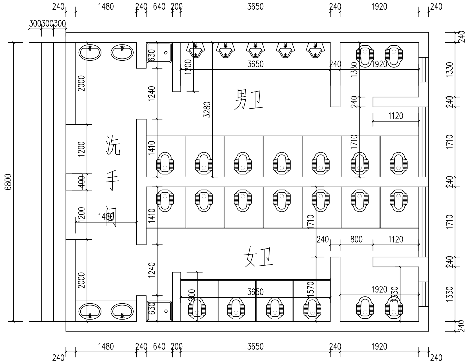
一楼男、女卫原平面图 1:50
