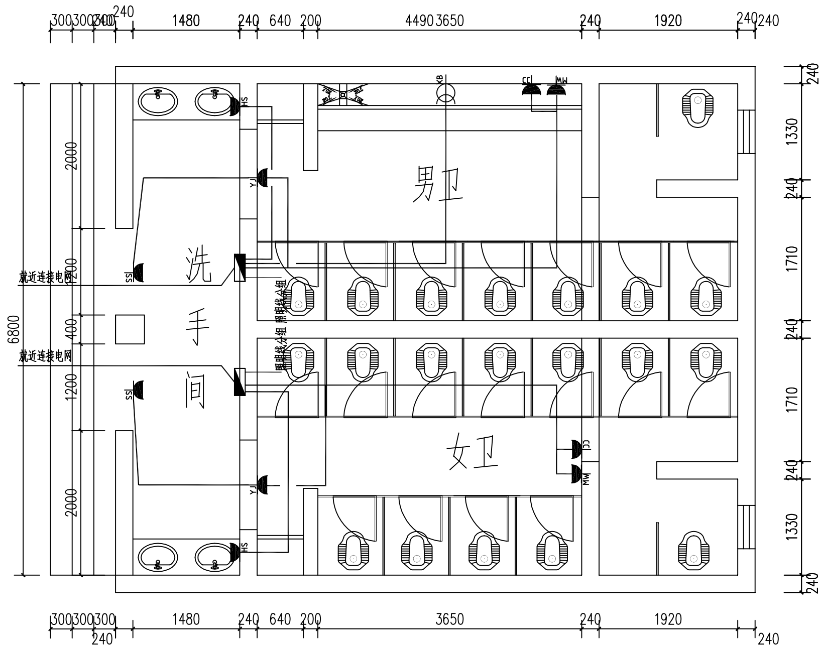
一楼男、女卫强电线路图 1:50
