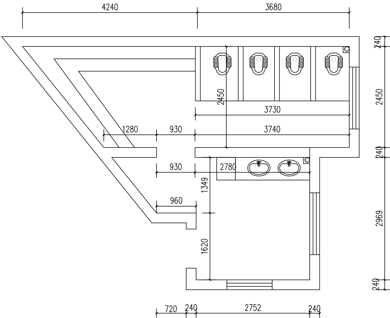
尚雅楼原男卫生间平面图 1:50
