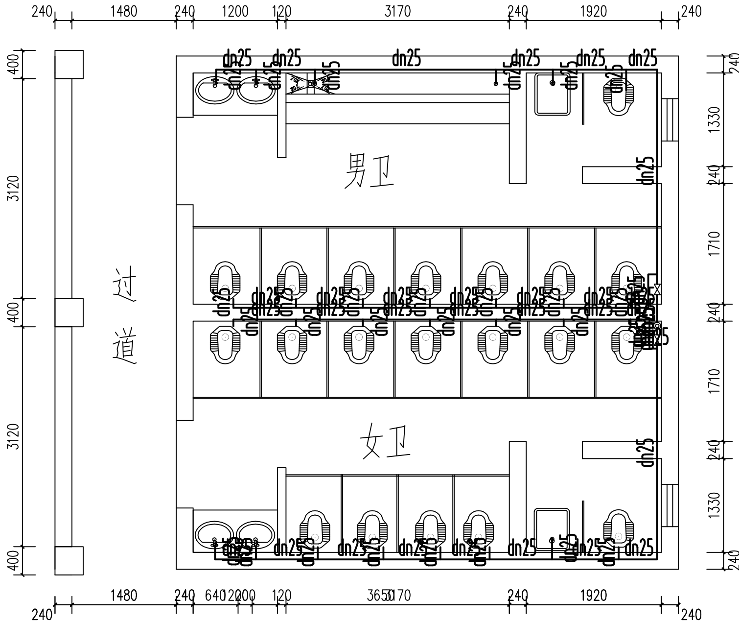
三楼男、女卫给水线路图 1:50
