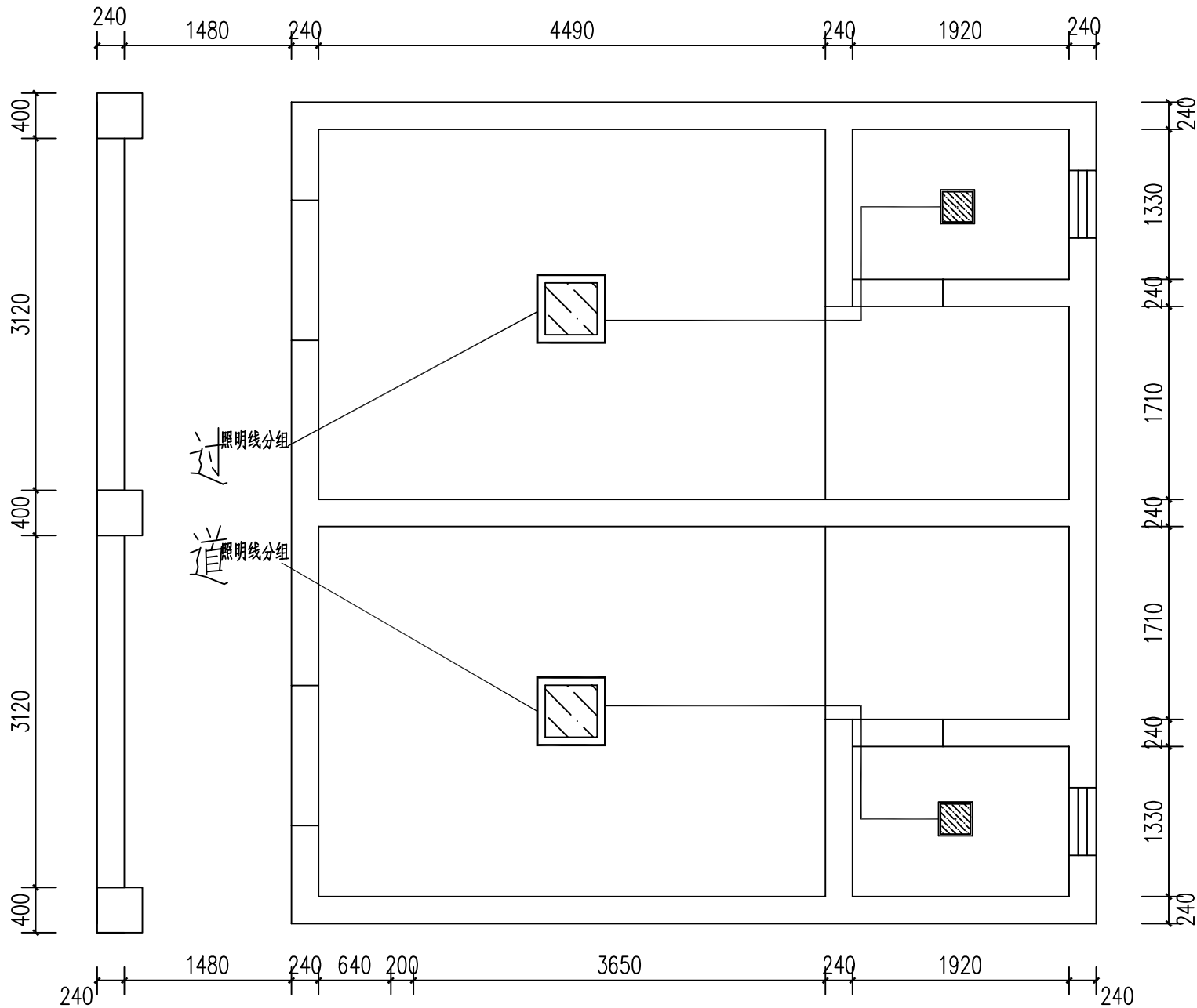
三楼男、女卫照明线路图 1:50
