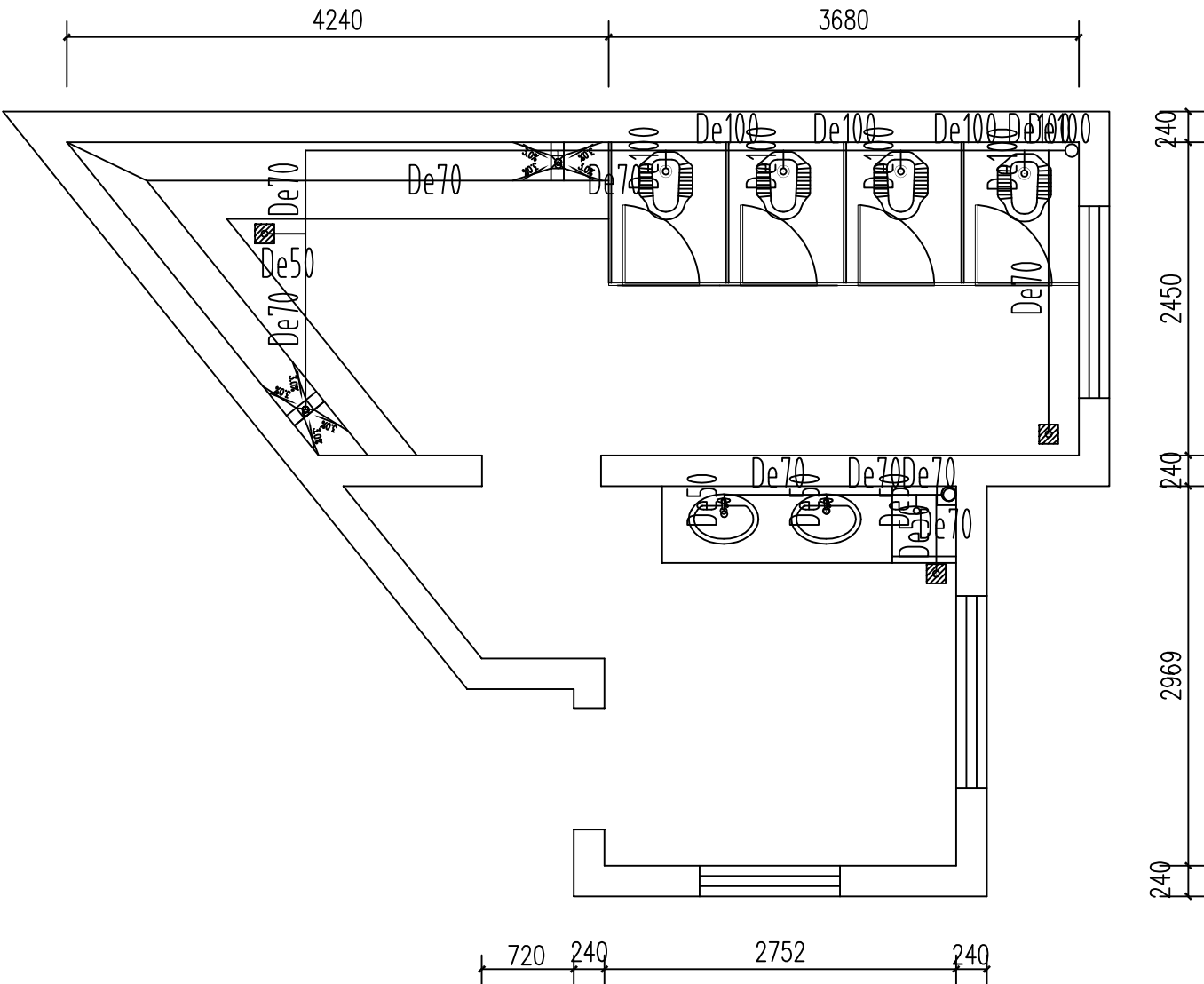
尚雅楼男卫生间排水线路图 1:50
