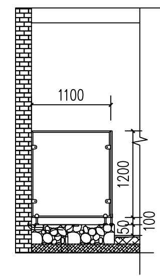
1-1剖面尺寸图
