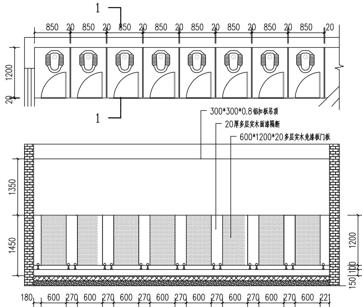
木质隔断立面尺寸图
