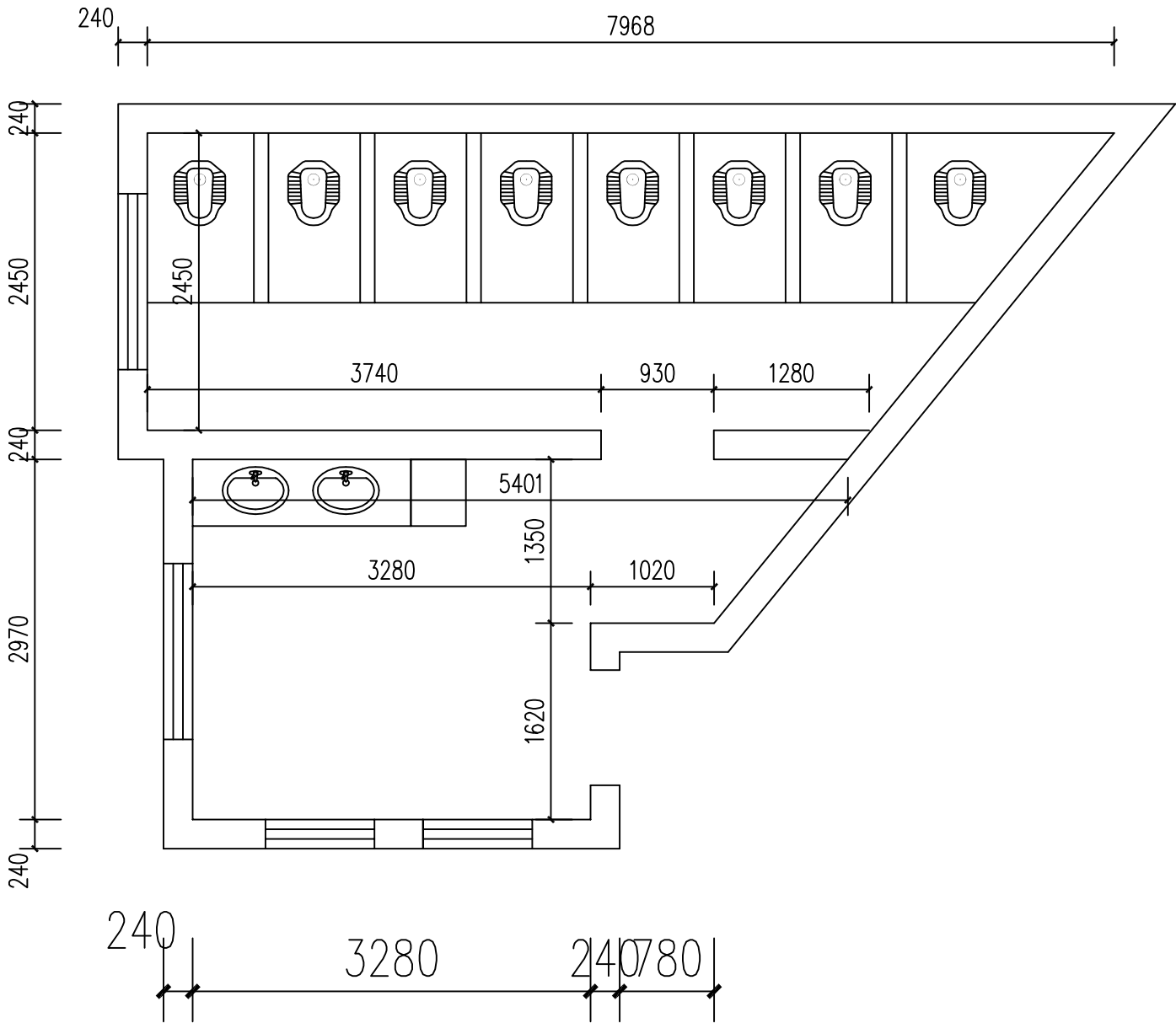
尚雅楼女卫生间拆除范围
