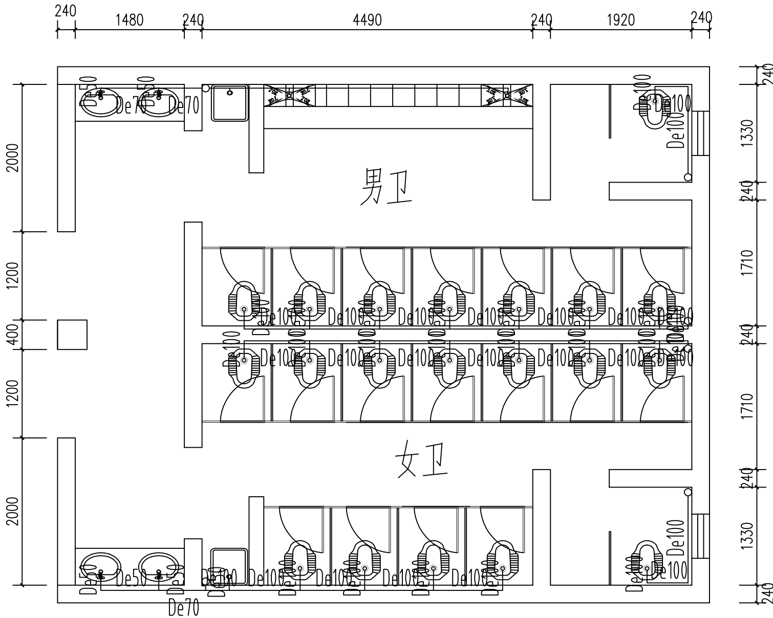
一楼男、女卫排水线路图 1:50
