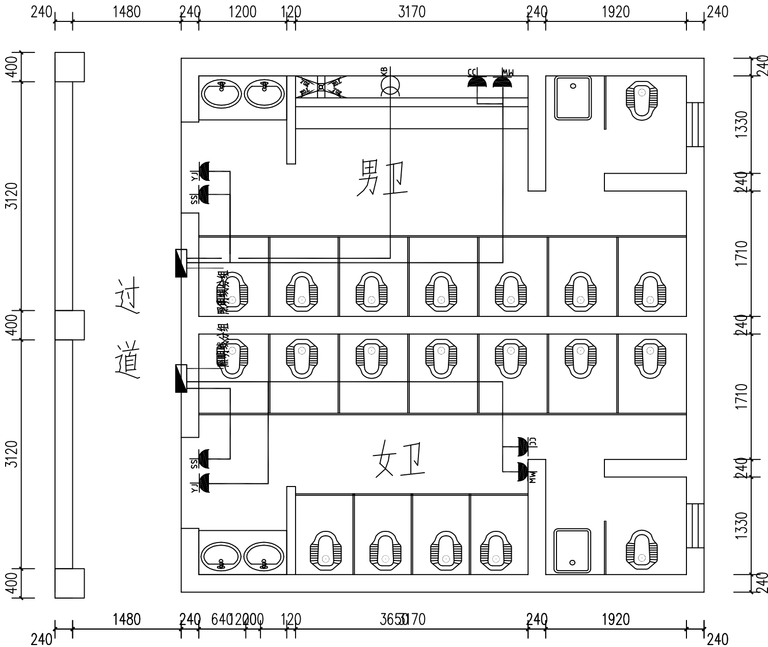
三楼男、女卫强电线路图 1:50
