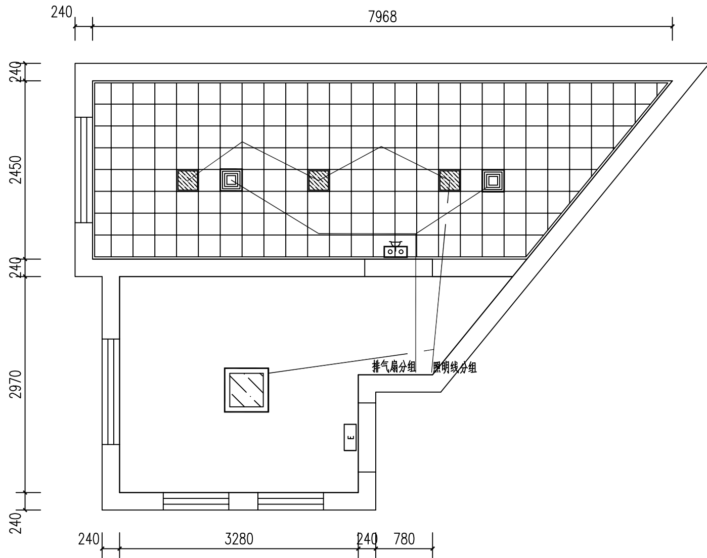
尚雅楼女卫生间照明线路图 1:50
