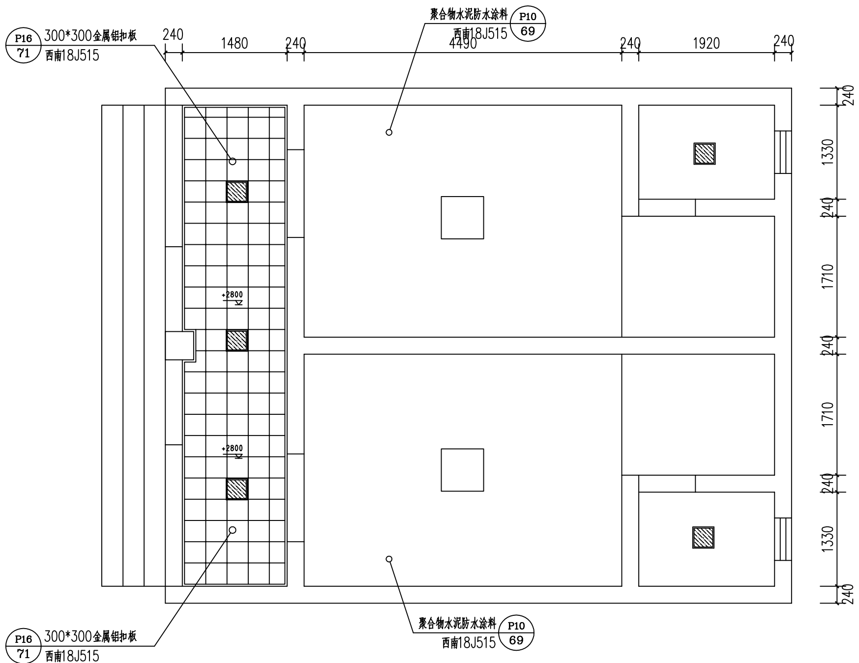
一楼男、女卫顶面材质图
