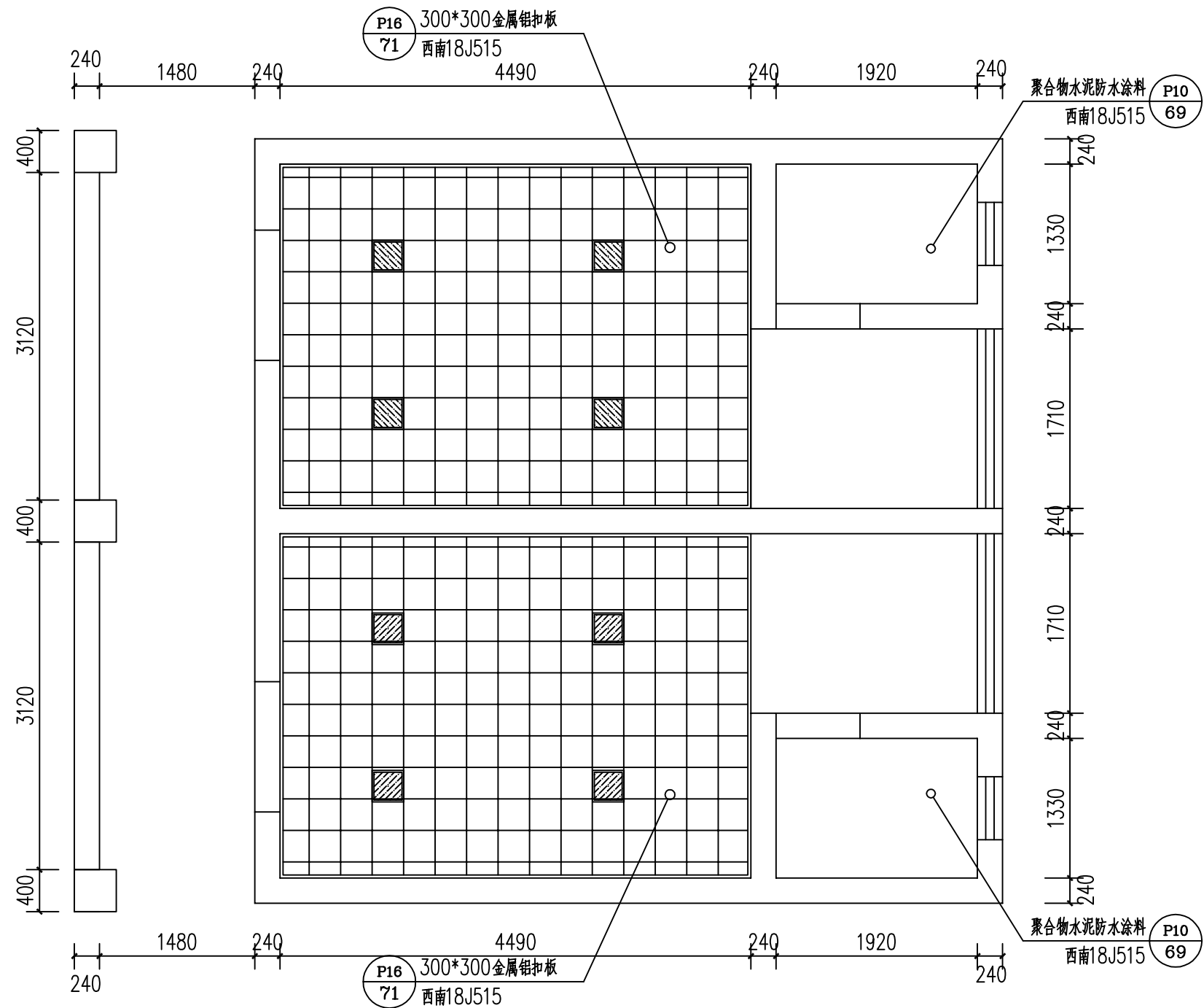
二楼监控室改造范围 1:50
