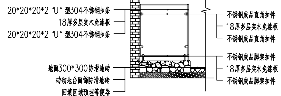
1-1剖面材质图
