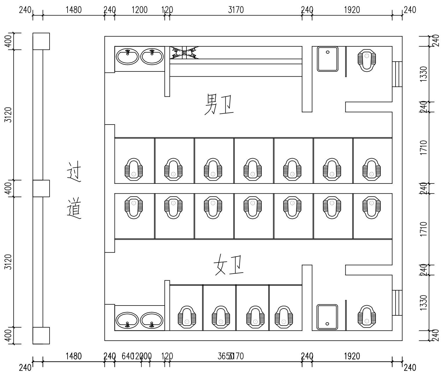
三楼男、女卫整改平面图
