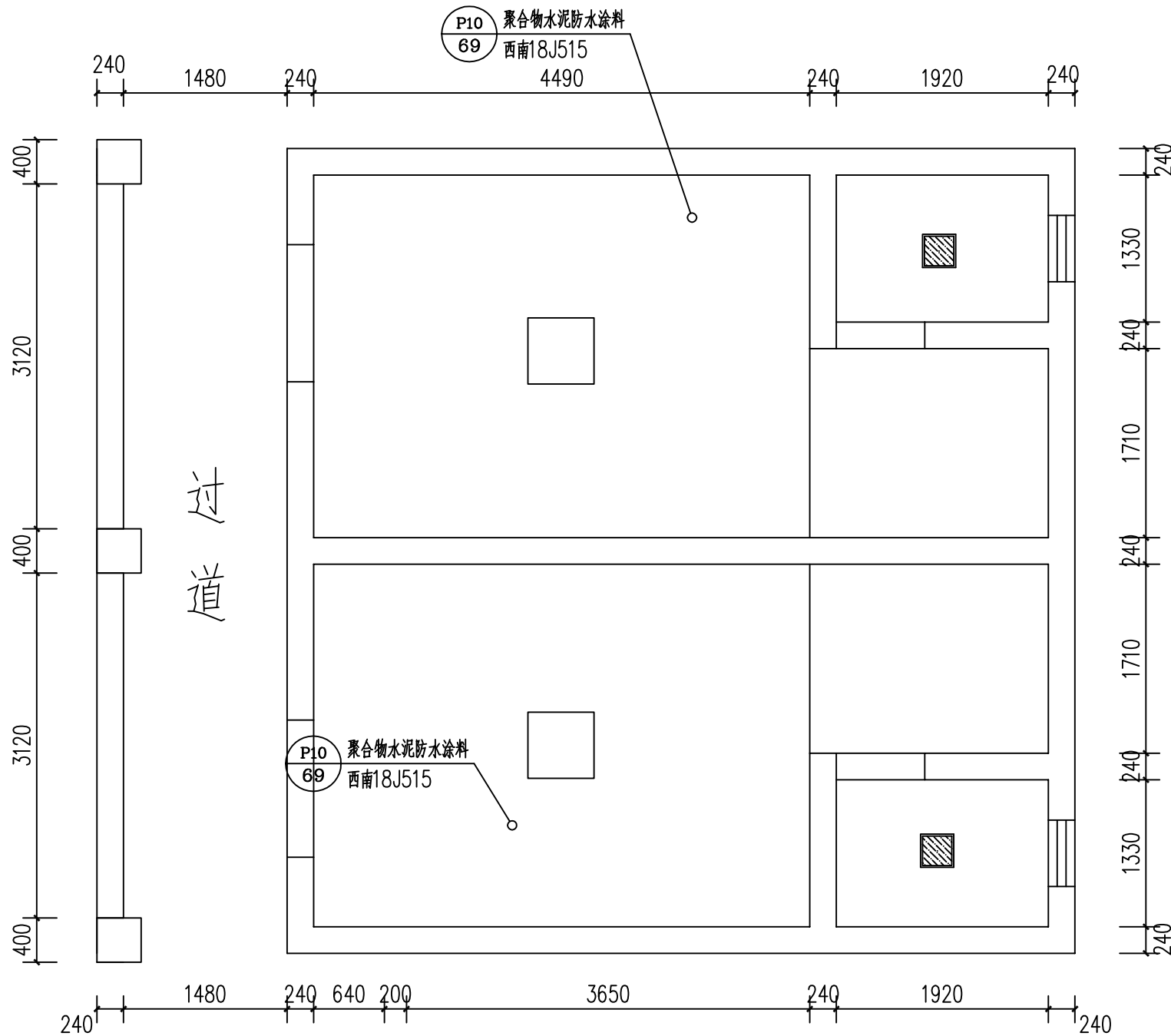
三楼男、女卫顶面材质图
