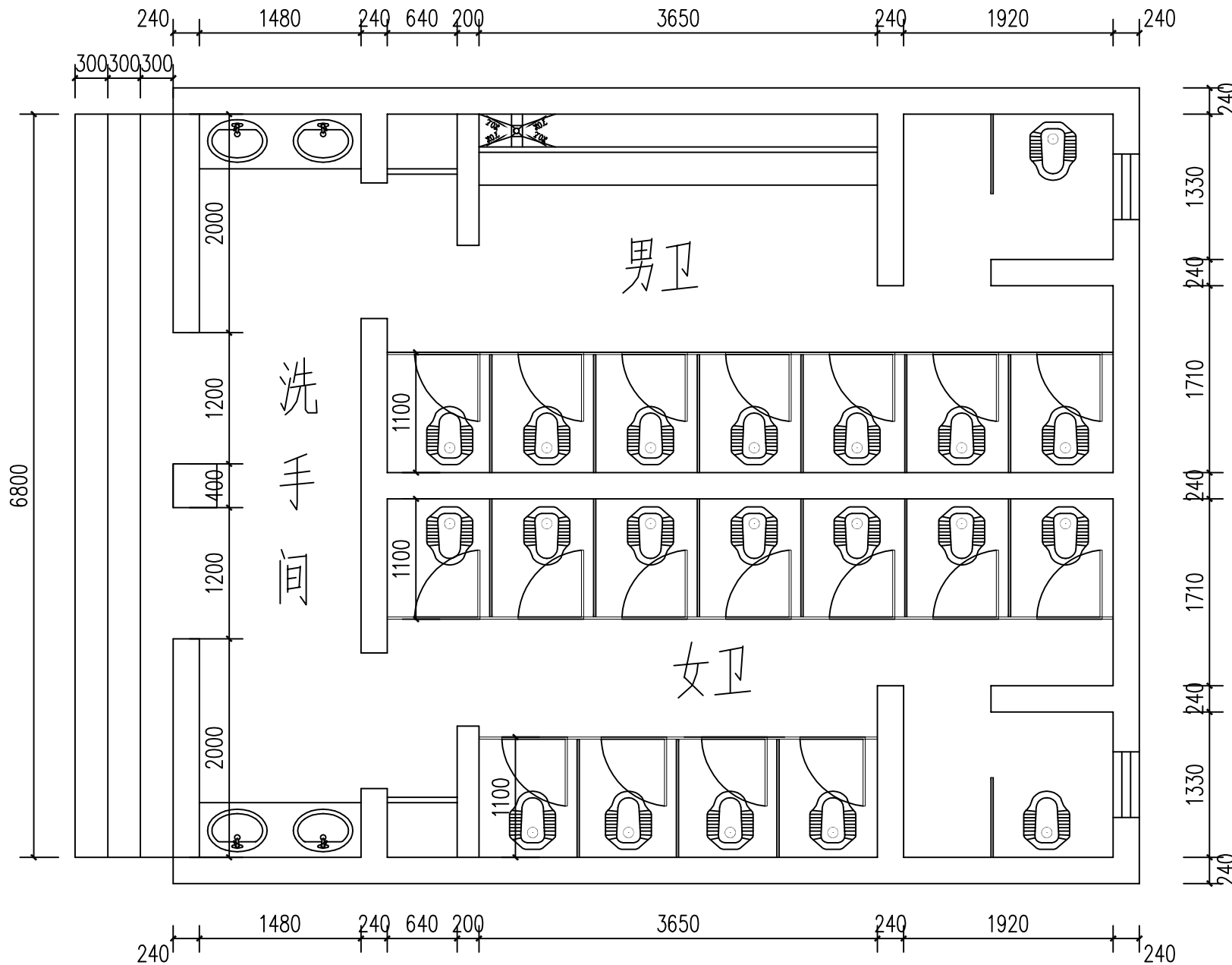
一楼男、女卫整改平面图
