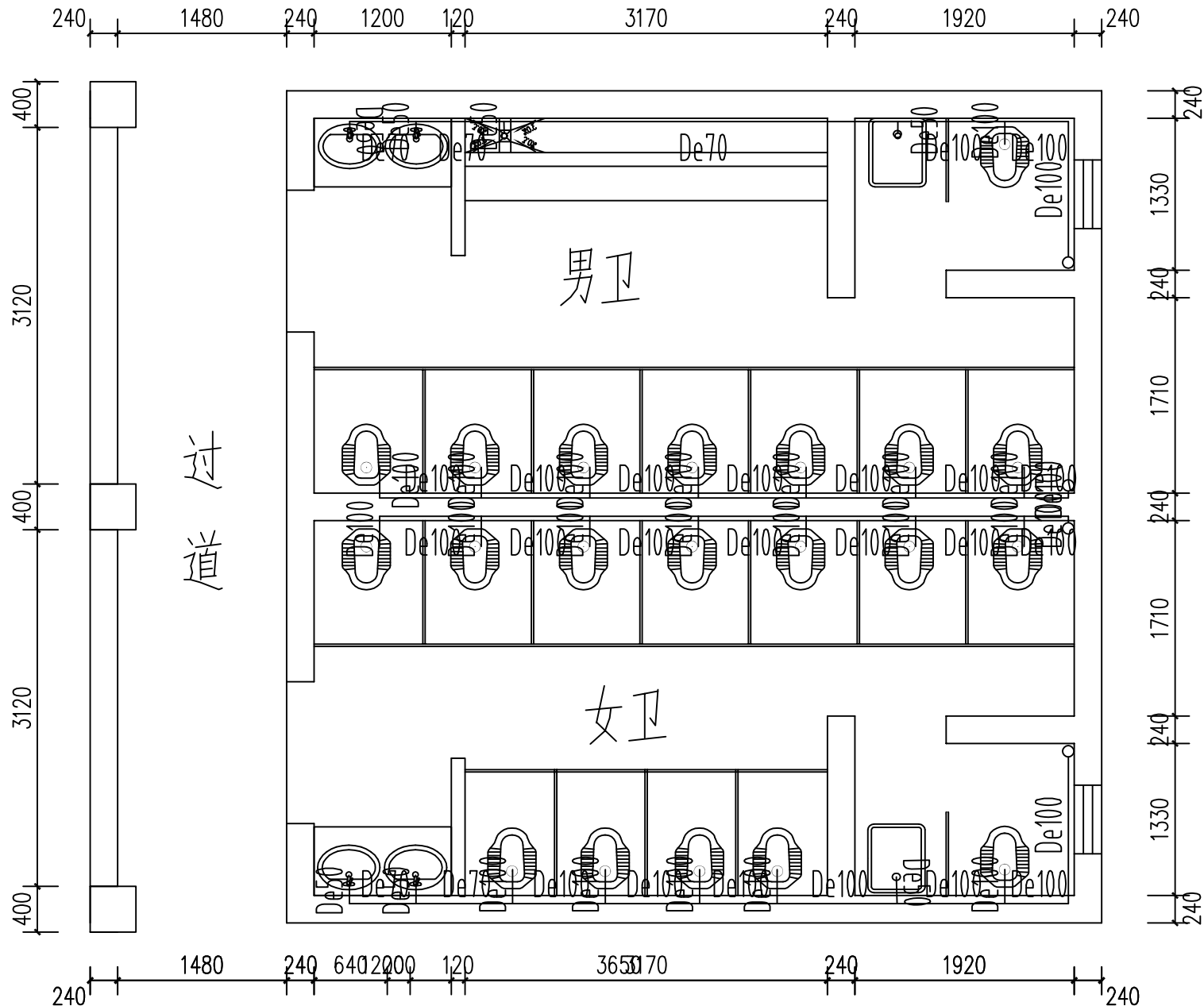
三楼男、女卫排水线路图 1:50
