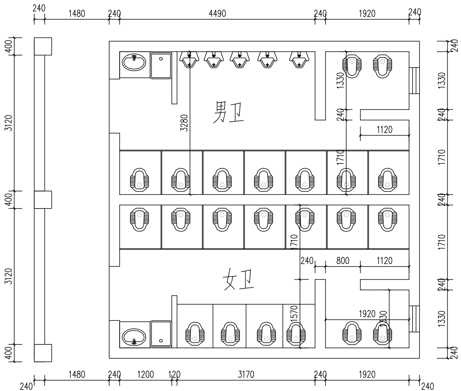
五楼男、女卫拆除范围 1:50
