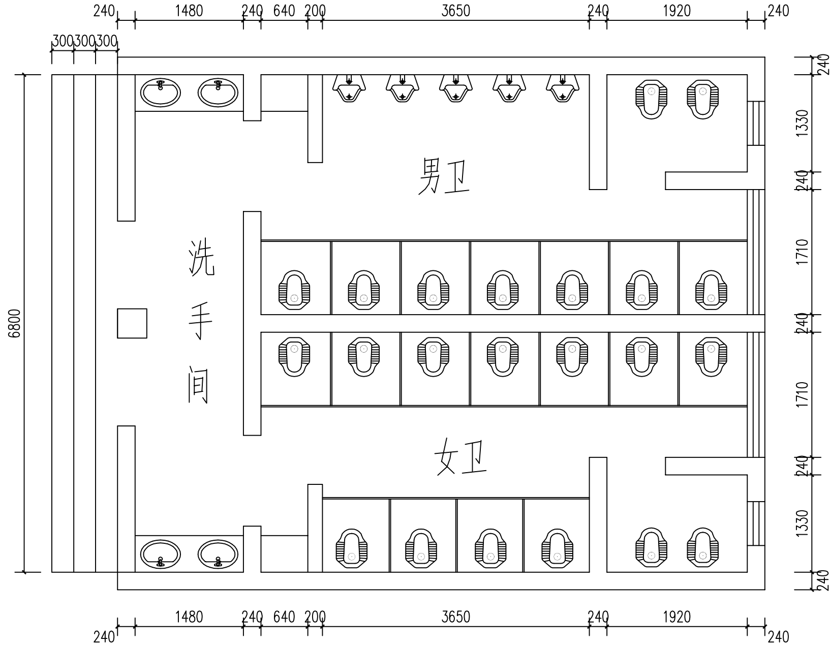
一楼男、女卫拆除范围 1:50
