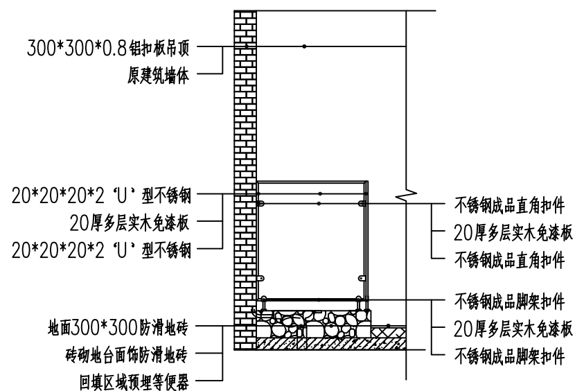
1-1剖面材质图
