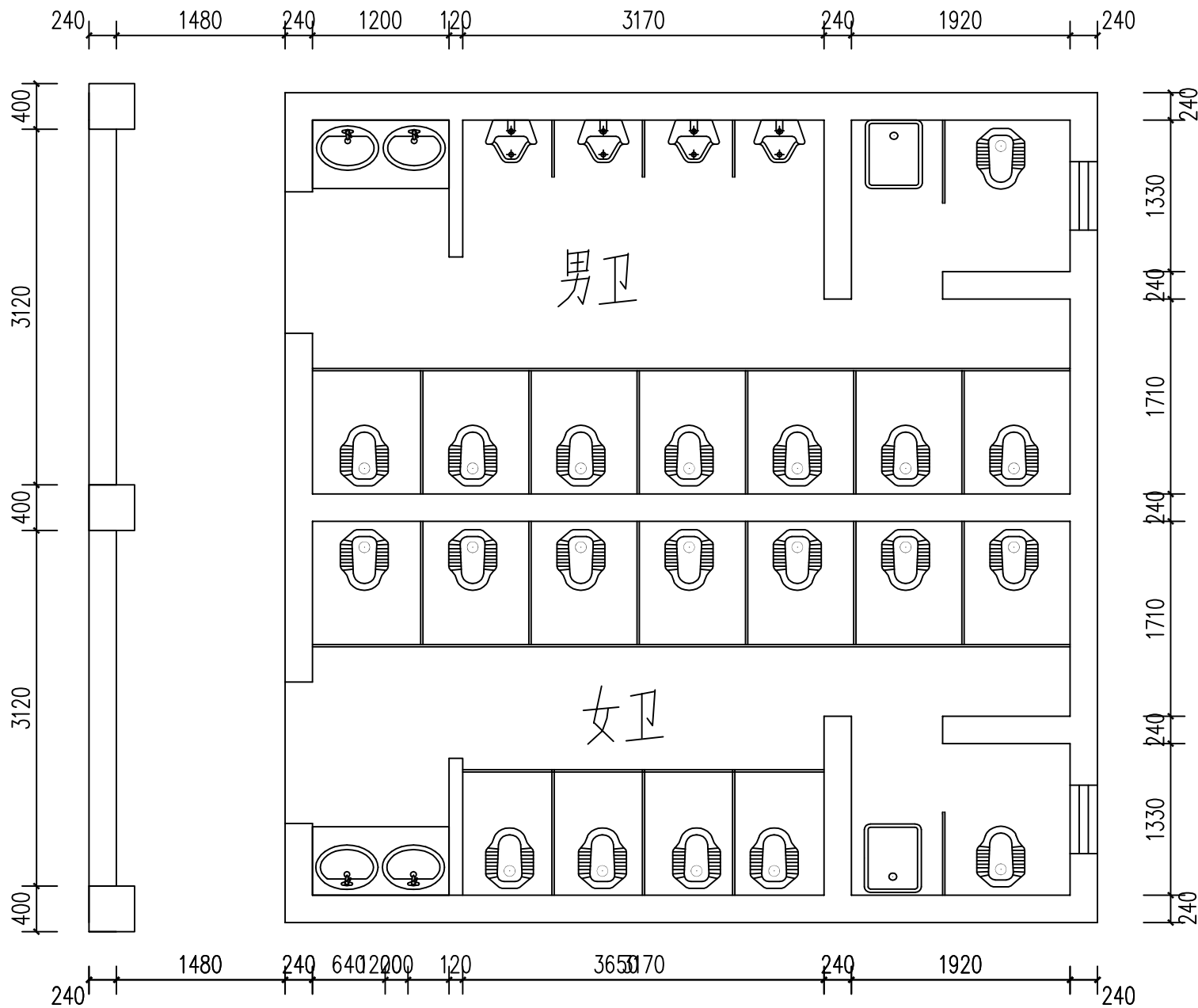
五楼男、女卫整改平面图
