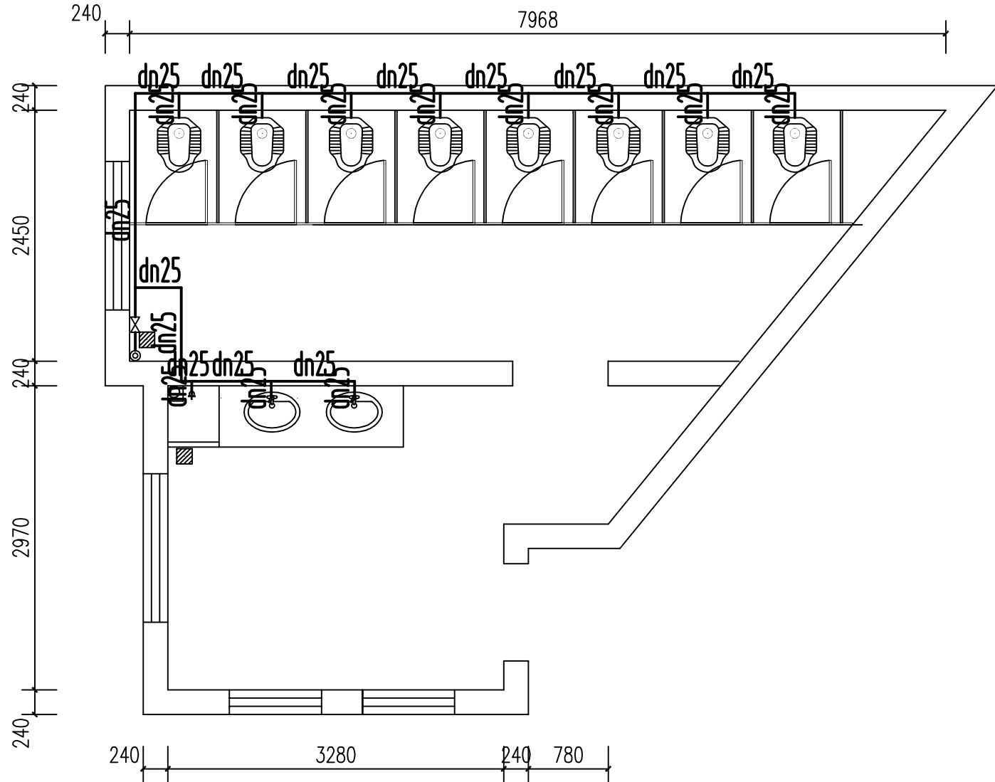
尚雅楼女卫生间给水线路图 1:50
