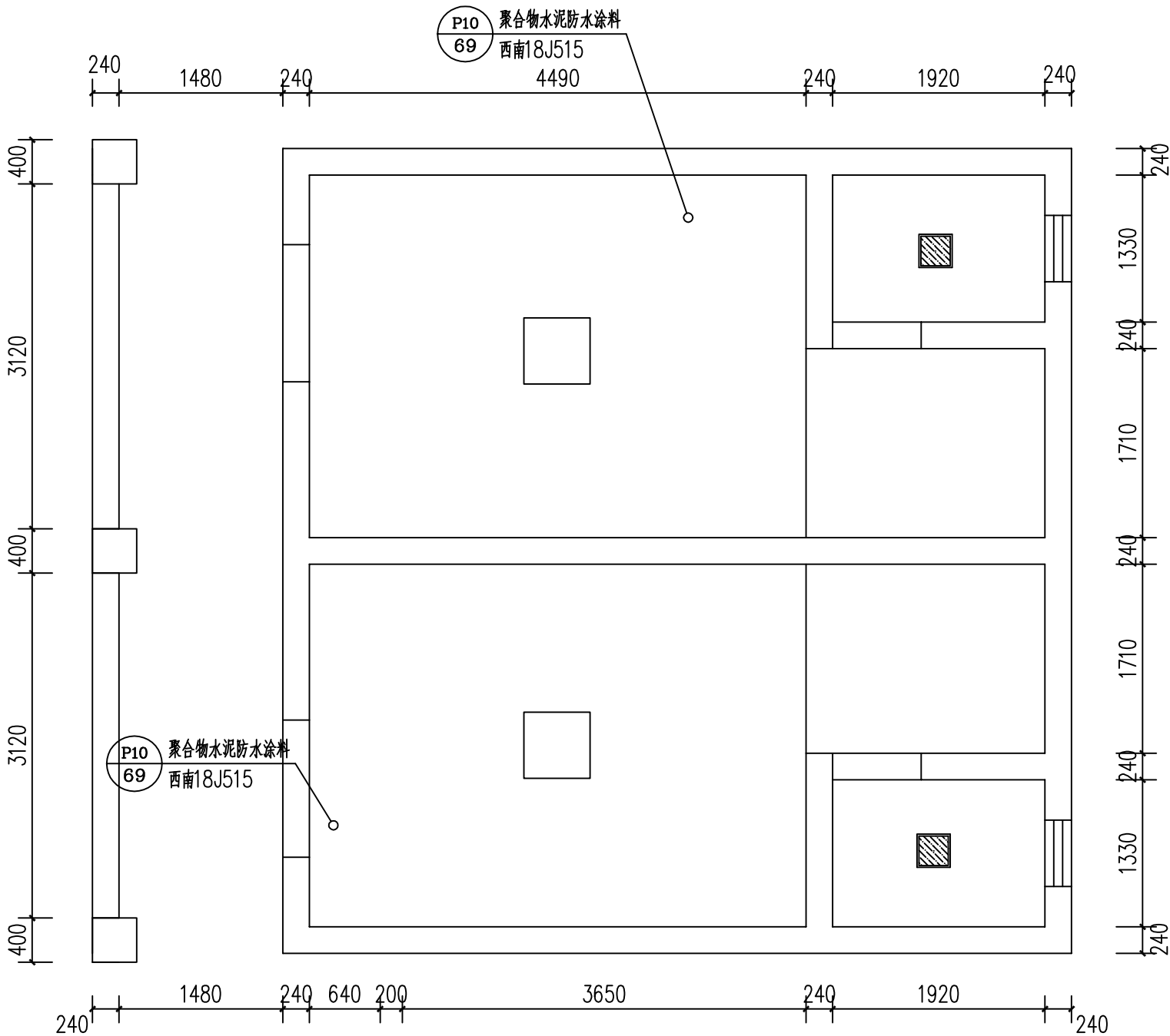
五楼男、女卫顶面材质图
