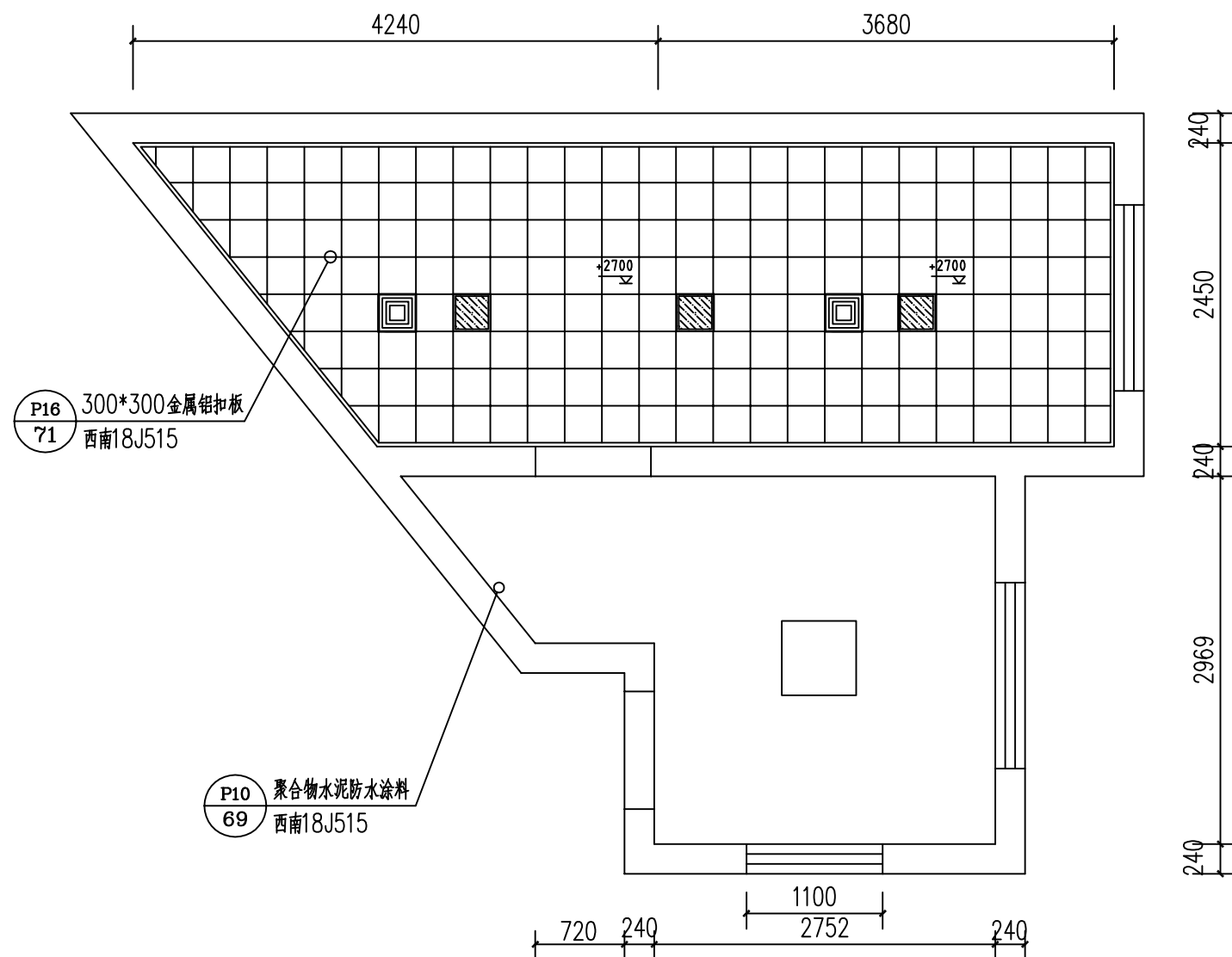
尚雅楼整改男卫生间吊顶图
