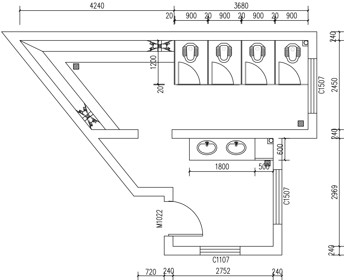
尚雅楼男卫整改平面图 1:50
