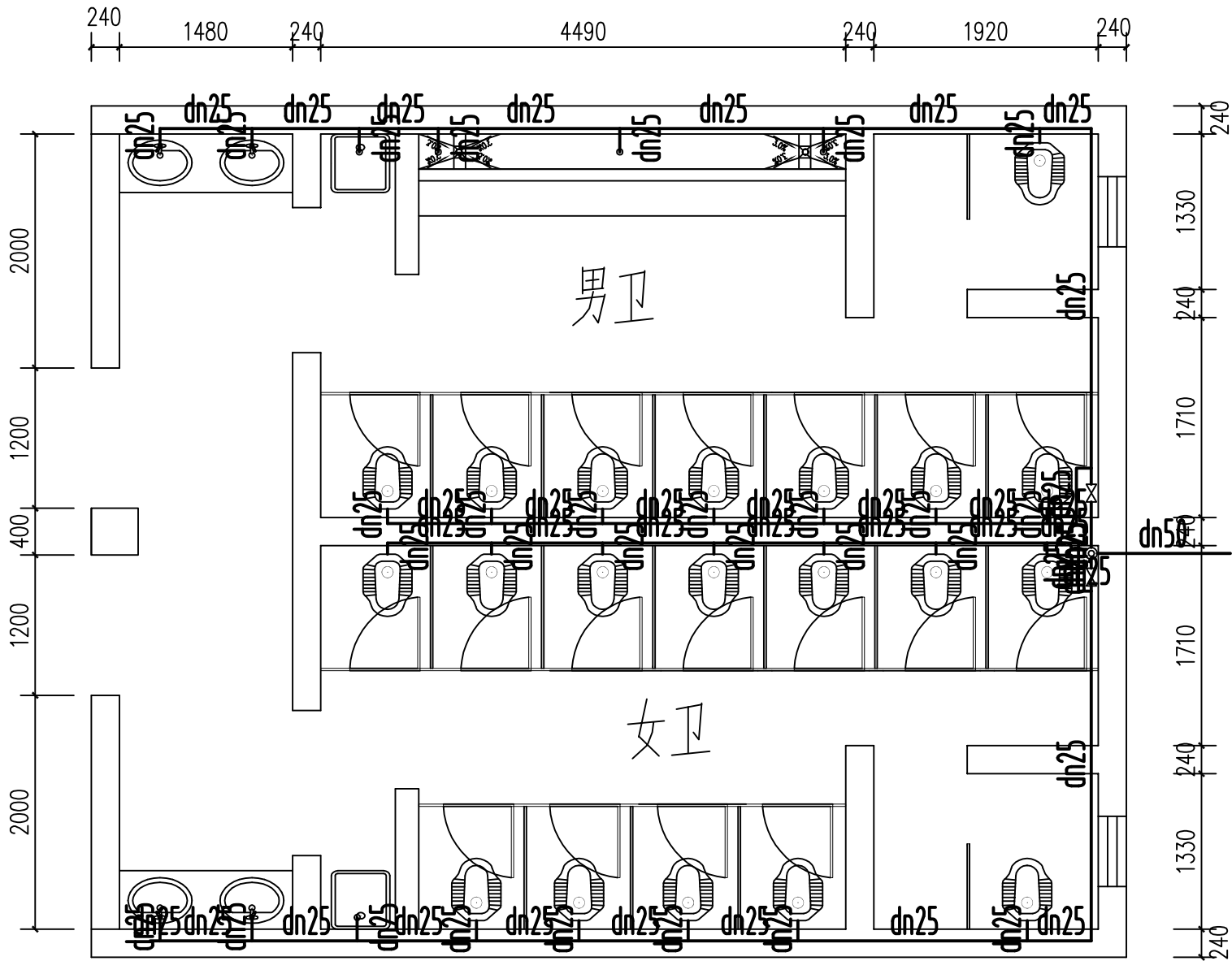
一楼男、女卫给水线路图 1:50
