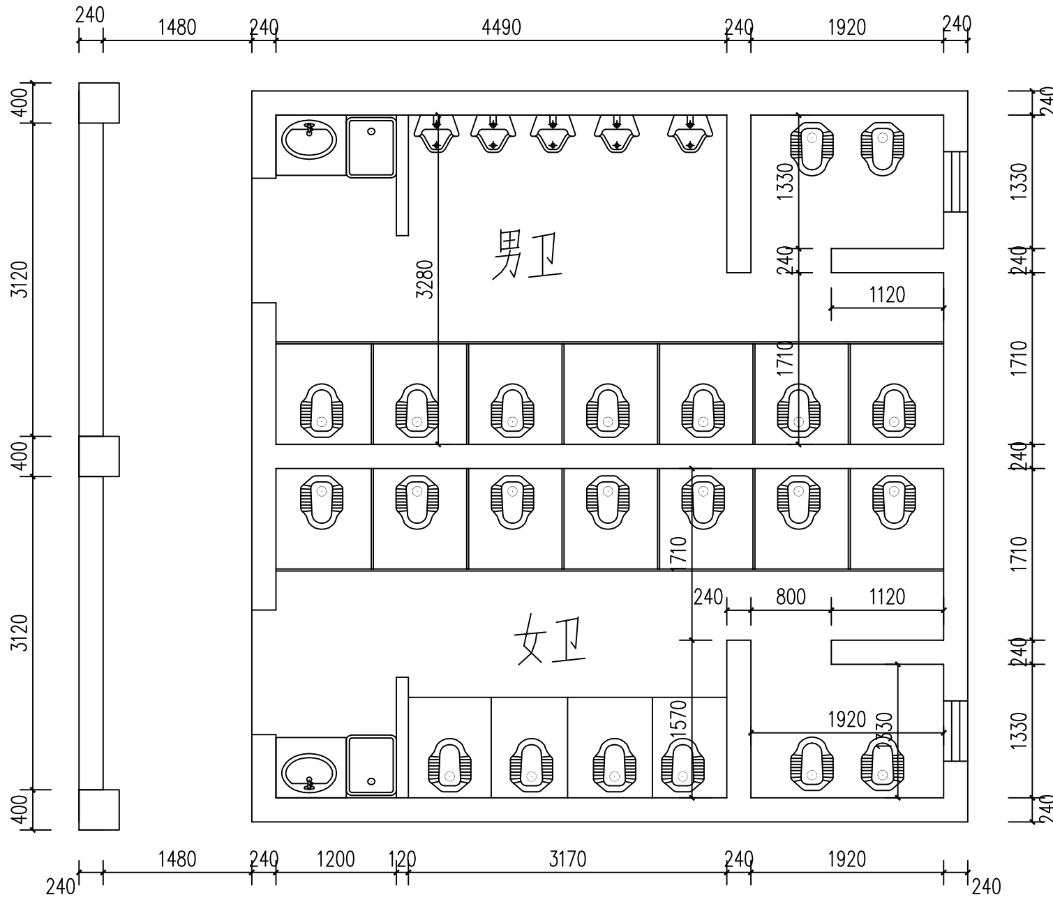
五原男、女卫平面图 1:50
