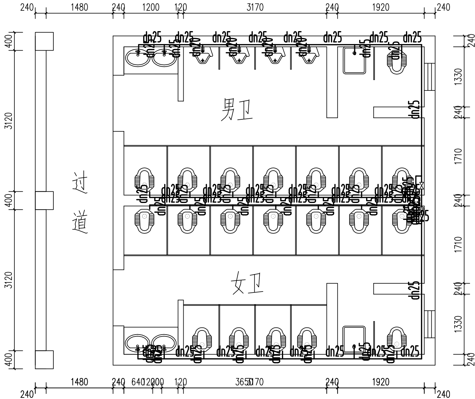
五楼男、女卫给水线路图 1:50
