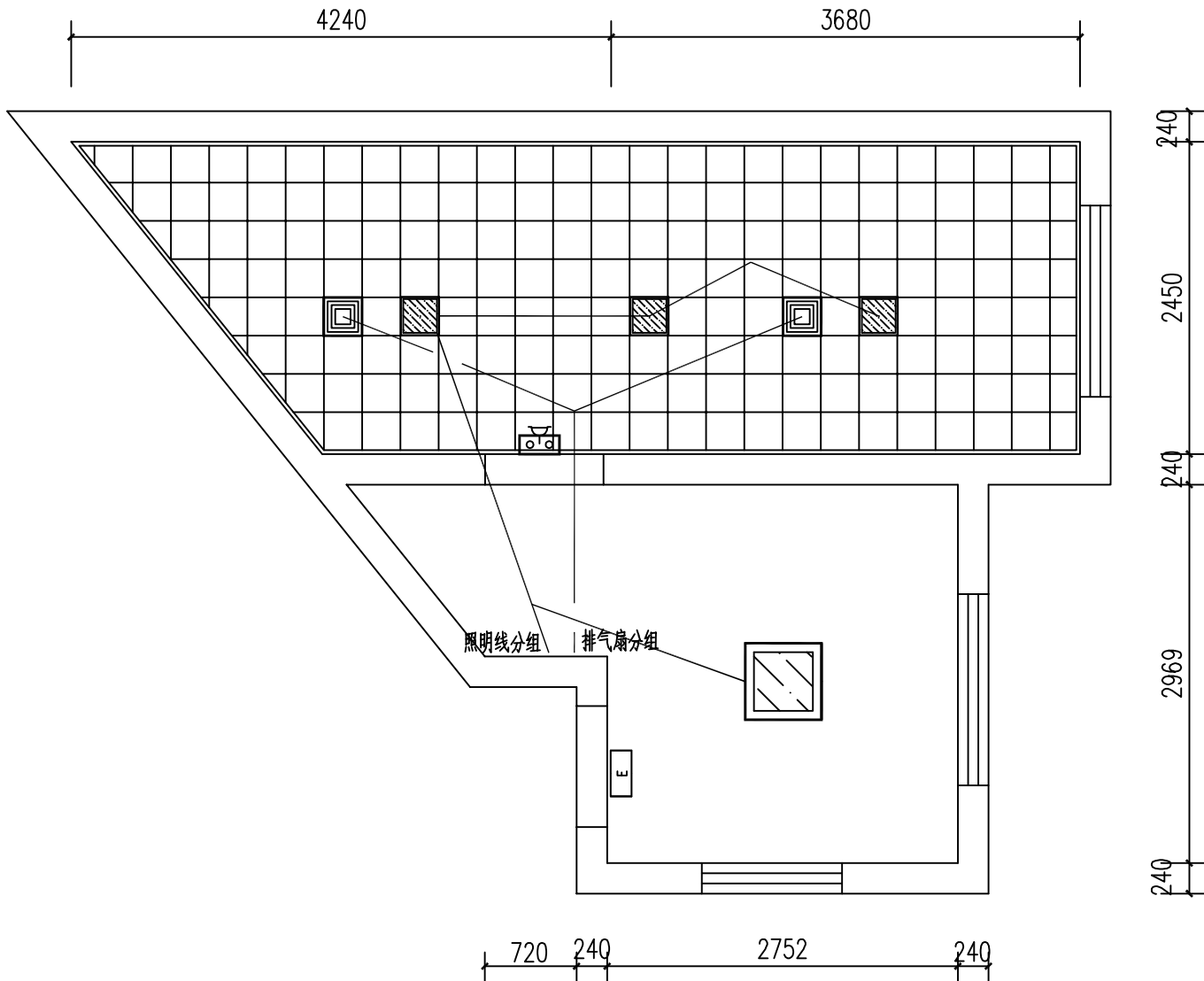
尚雅楼男卫生间照明线路图 1:50
