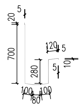
不锈钢小便槽大样
