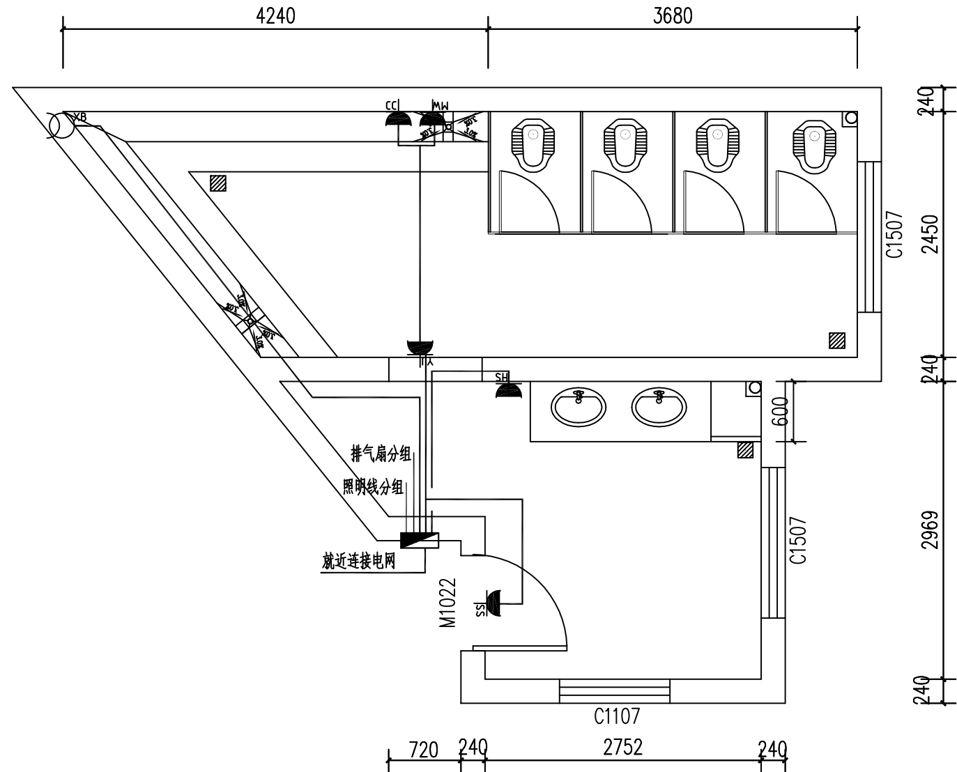
尚雅楼男卫生间强电线路图 1:50
