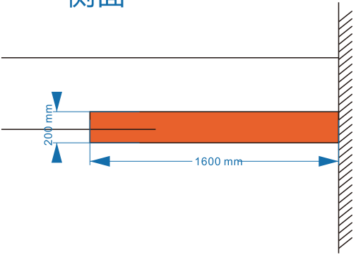
侧面
