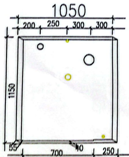
厕所花纹钢底板及开孔平面图
