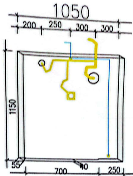
厕所花纹钢底板及开孔平面图
