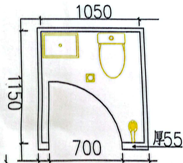
图中尺寸皆为内空尺寸
